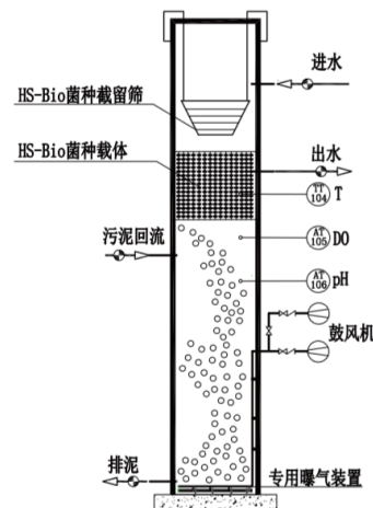
HS-Bio高盐有机废水生化反应器示意图
